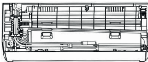
Entwässerungsanschlüsse
